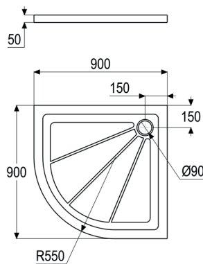
Z055311-00000 Duschwanne halbrund ST 1009 Farbe grau Werkstoff kalkhaltiger Naturstein
