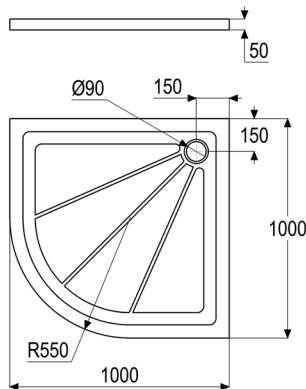
Z055310-00000 Duschwanne halbrund ST 1000 Farbe grau Werkstoff kalkhaltiger Naturstein
