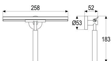
Z043880-00010 Duschwischer chrom Griff chrom Wandhalter chrom Wischerlippe grau Wandmontage mit Wandbefestigung
