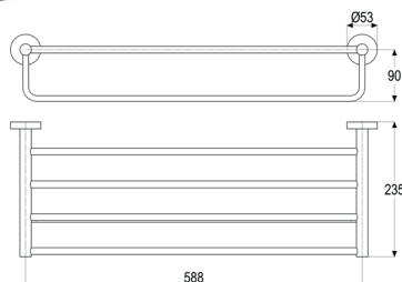
Z043189-00010 Handtuchablage chrom Länge 600 mm mit Badetuchhalter Wandmontage mit Wandbefestigung
