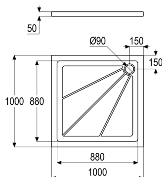
Z055320-00000 Duschwanne eckig ST 3000 Farbe grau Werkstoff kalkhaltiger Naturstein
